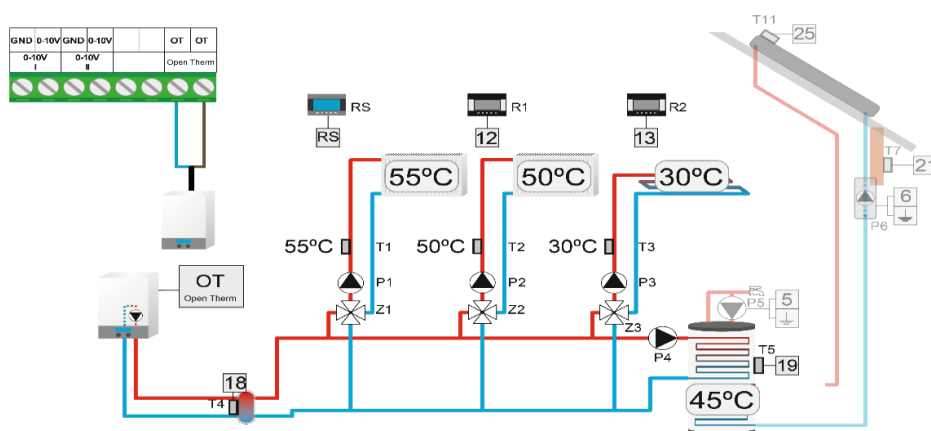
Příklad zapojení instalace Open Therm
