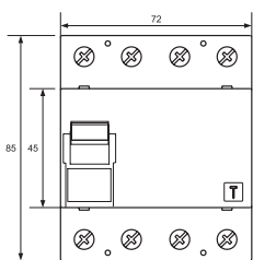
DFS 4 B – rozměry, schéma zapojení
