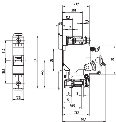
DUSA – rozměry, schéma zapojení
