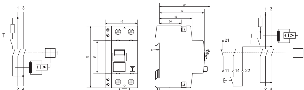
DFS 2 AC FT / A FT – rozměry, schéma zapojení
