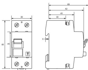
DFS 2 AC / A / A KV / AC S / A S – rozměry, schéma zapojení
