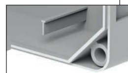
Speciálně tvarovaná stěna víka a tím dosažení mechanické odolnosti na hodnotu IK08
