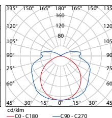
DUST EVG PC 2 ×36W
