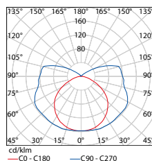
DUST EVG PC 1 ×36W
