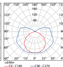
DUST EVG PC 1 ×58W
