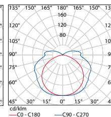
DUST EVG PC 2 ×58W
