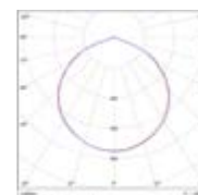
GULIVER AL 115 reflektor
