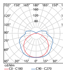
TRUST EVG PC 2 ×36W
