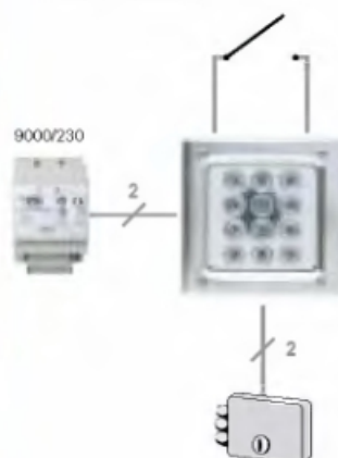
Kódová klávesnice
