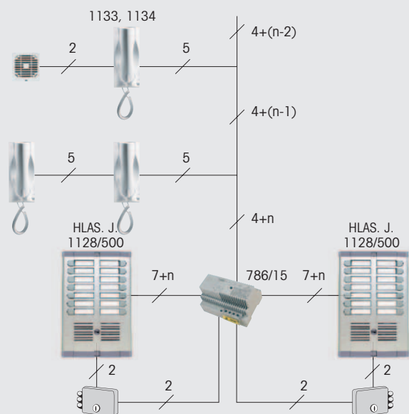
Komunikace s automatickým přepínáním 2 tlačítkových panelů
