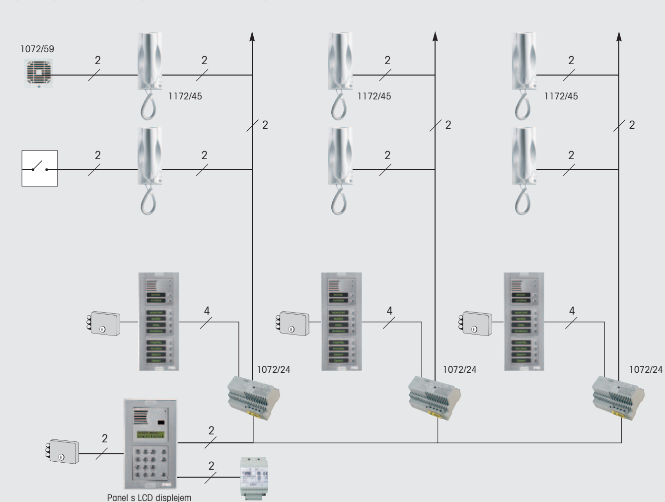
Digitální systém 1072. Zapojení 1 hlavní a X podružných vstupů.
