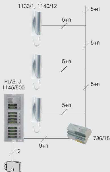
Komunikace s tlačítkovým panelem a interkomová funkce mezi účastníky
