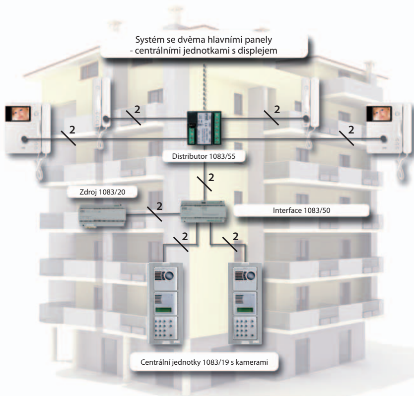
Více objektů se společným hlavním vstupem
