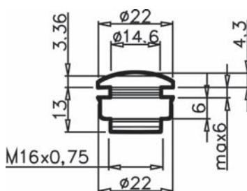
Rozměry PROTACT
