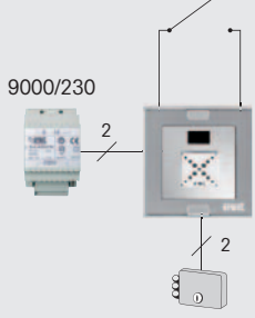
Snímač elektronických klíčů 1148/45
