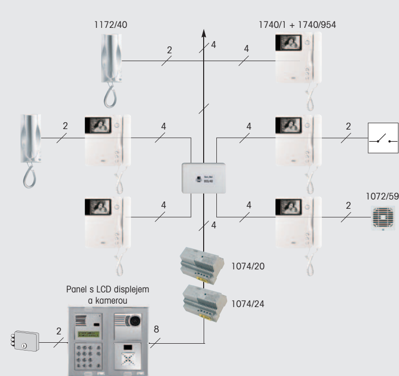
Digitální systém 1072. Kombinace telefonů a videotelefonů.
