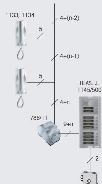
Komunikace s tlačítkovým panelem
