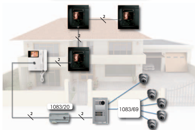
Systém s jedním vstupním tablem - připojení externích kamer
