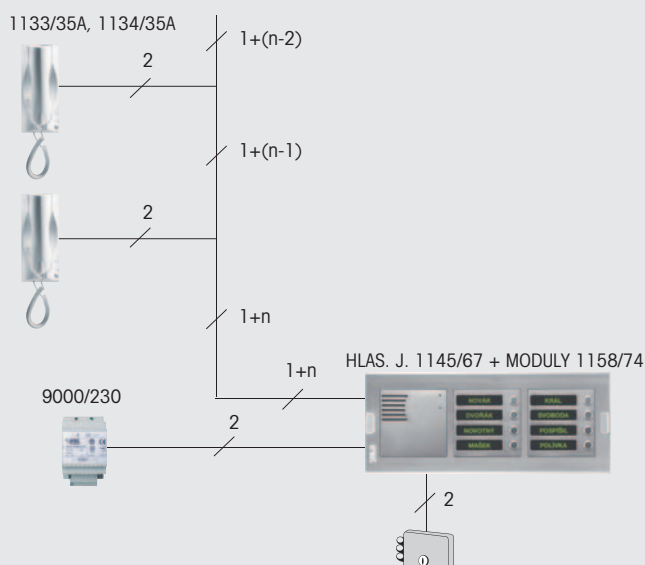
Komunikace s tlačítkovým panelem (1+n)
