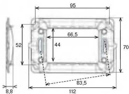
obdélníkový montážní rámeček 3 moduly
