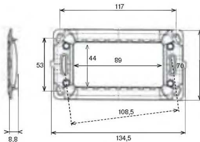
obdélníkový montážní rámeček 4 moduly
