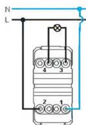
dvupólový spínač (řazení 2)
