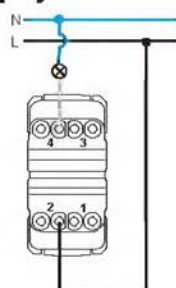
jednopolový spínač (řazení 1)
