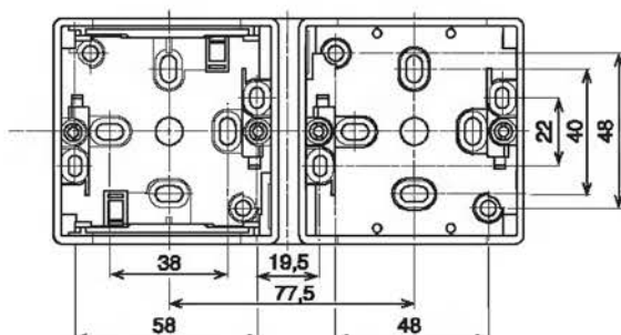
monoblokové vodotěsné pouzdro
