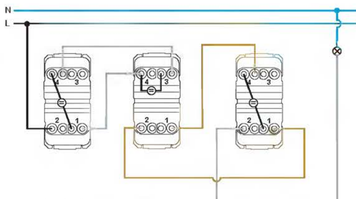
2 střídavé přepínače + 1 křížový přepínač s orientační kontrolkou
