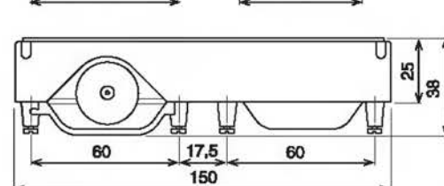
horizontální dvojité krabice
