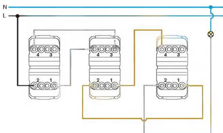
2 střídavé přepínače + 1 křížový přepínač
