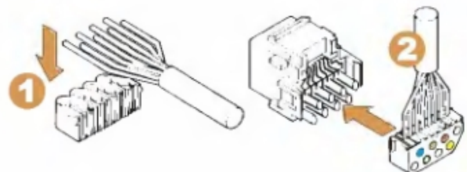
způsob bezšroubového připojení
