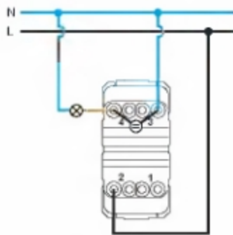
jednopolový spínač se signalizační kontrolkou
