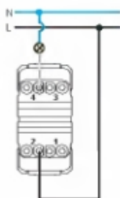
jednopolový spínač (řazení 1)
