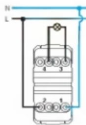
dvojpolový spínač (řazení 2)
