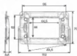
obdélníkový montážní rámeček 2 otvory
