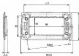
obdélníkový montážní rámeček 4 otvory
