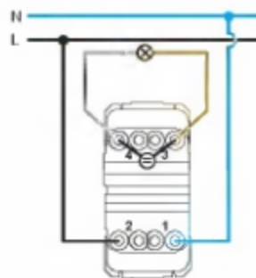
dvoupólový spínač s kontrolkou
