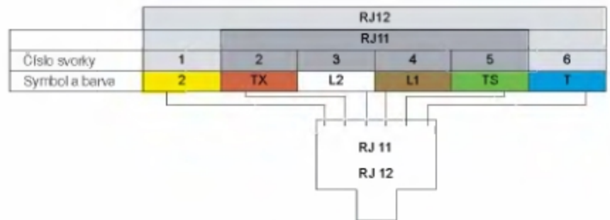
způsob bezšroubového připojení
