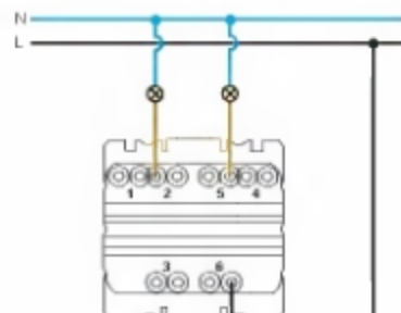
sériový přepínač (řazení 5)
