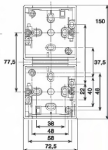
vertikální dvojitá krabice
