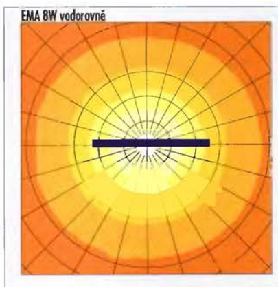
osvětlenost/luminosity (lx) 950x850mm
