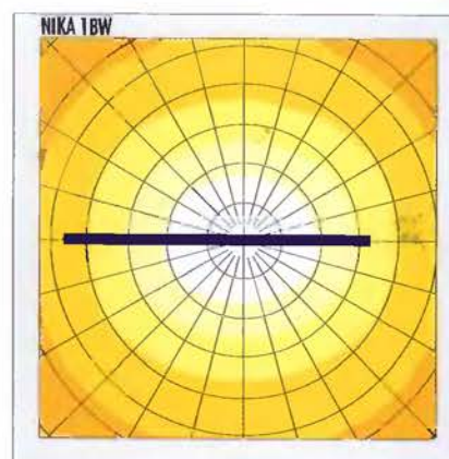
NIKA 1BW osvětlenost/luminosity (lx) 900x1000mm
