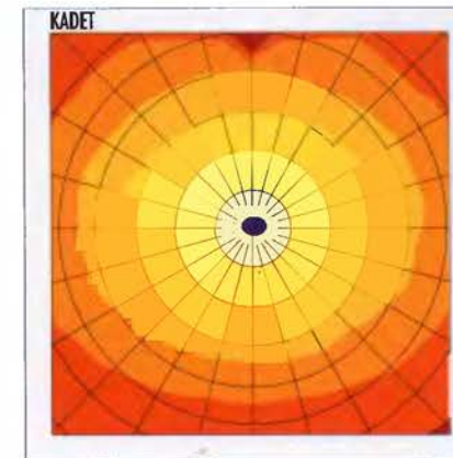
osvětlenost/luminosity (lx) 1000x950mm
