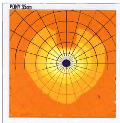
PONY 35cm osvětlenost/luminosity (lx) 900x950mm
