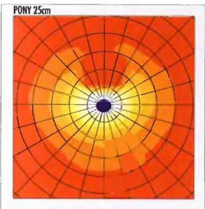
PONY 25cm osvětlenost/luminosity (lx) 800x800mm
