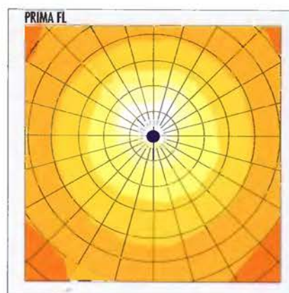
PRIMA FL osvětlenost/luminosity (lx) 1000-850mm
