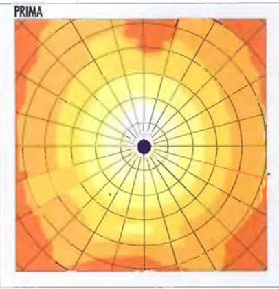
osvětlenost/luminosity (lx) 1000x900mm
