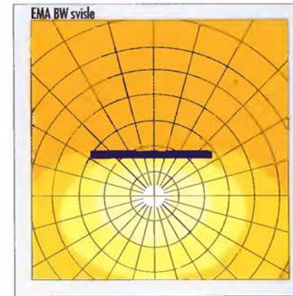
osvětlenost/luminosity (lx) 850x500mm
