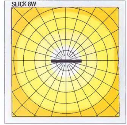
osvětlenost/luminosity (lx) 950x1000mm
