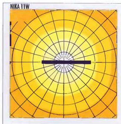
NIKA 11W osvětlenost/luminosity (lx) 850x1050mm
