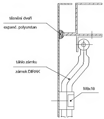
Detail těsnění dveří
