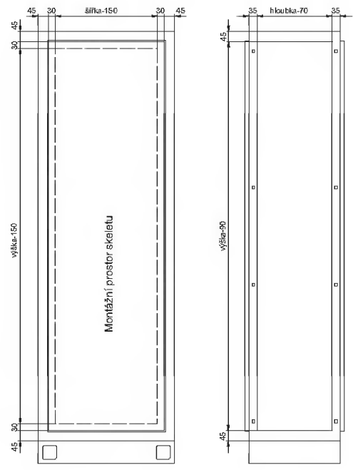
Skříň bez krytů
