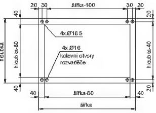
Pohled ze spodu na podstavec
