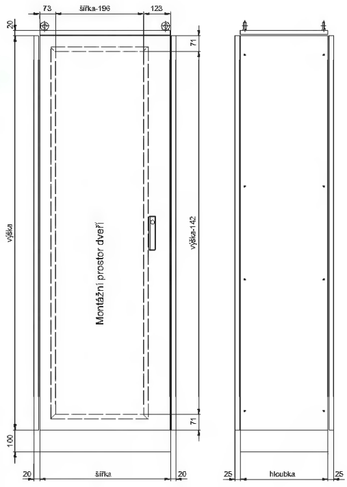
Skříň s kryty
