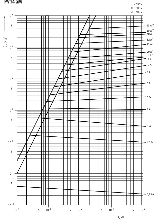
Charakteristika I^2t_a PV14 aM
