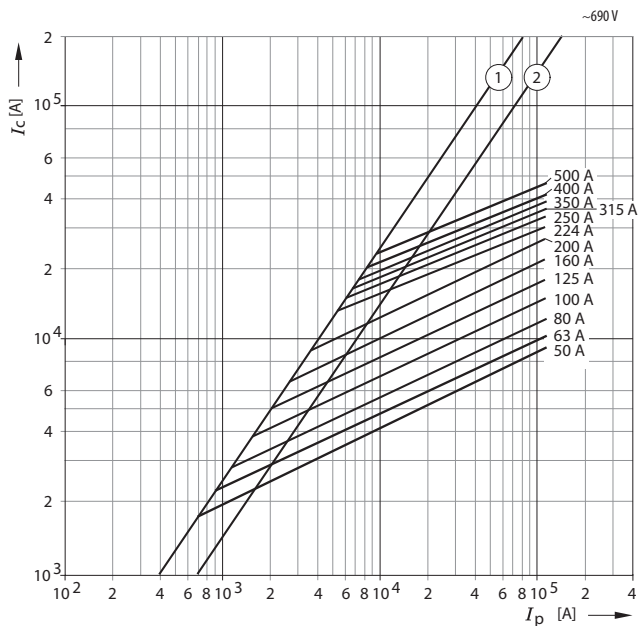
Omezovací charakteristika PHNA1, 2, 3 gG
