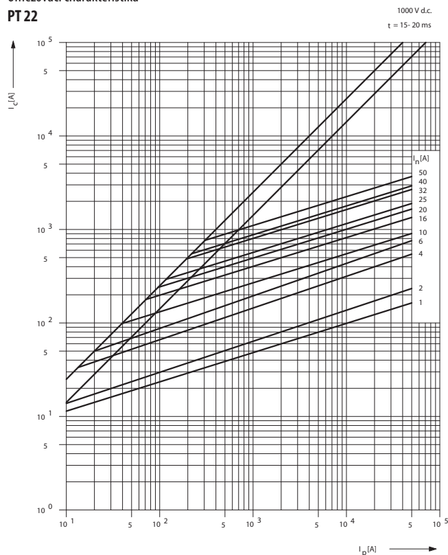
Omezovací charakteristika
