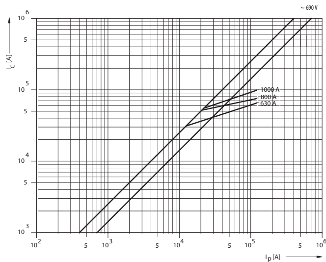
Omezovací charakteristika PHN4a gG
