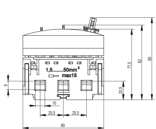
FH000-3A/T a FH000-3L/T
