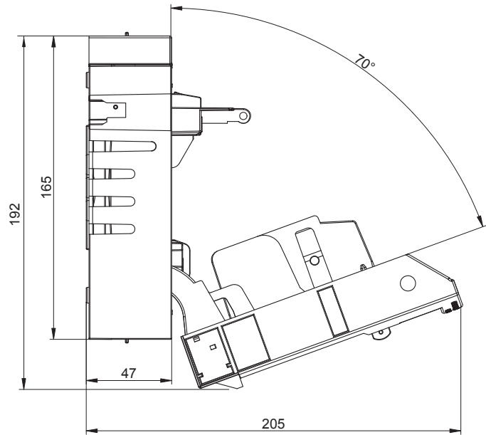
Odpínače FH00-3S/F a FH00-1S/F v otevřené poloze
