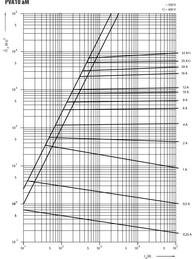
Charakteristika I^2t_a PVA10 aM
