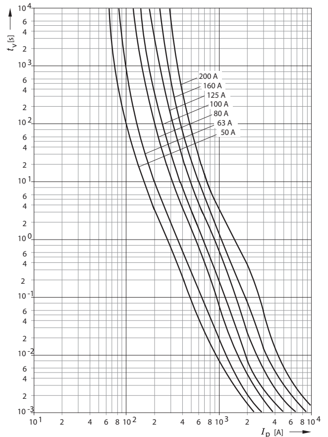
Tavná ampérsekundová charakteristika PHNA1 gG
