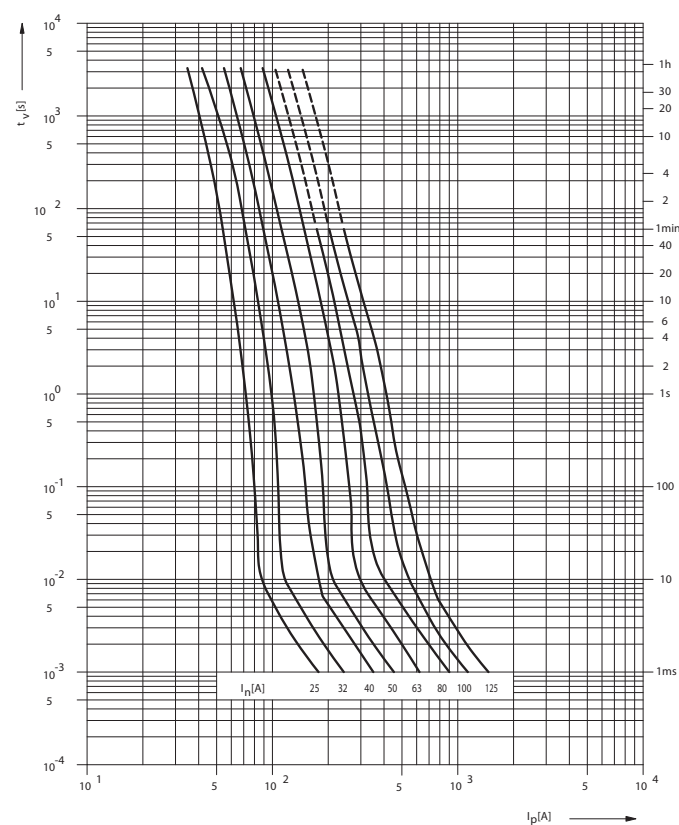
Tavná ampérsekundová charakteristika P50N06 gR, aR
