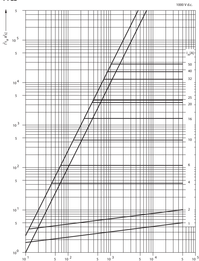
Charakteristika I^2t_a
