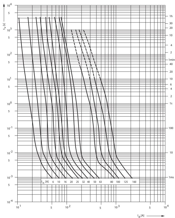
Ťavná ampérsekundová charakteristika P51R06 gR, aR
