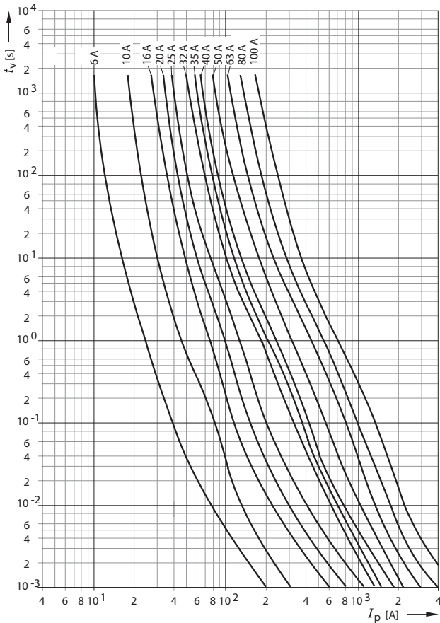
Tavná ampérsekundová charakteristika PHNA000, 00 gG
