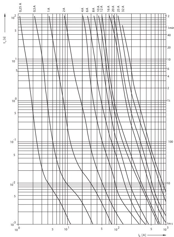
Tavná ampérsekundová charakteristika PVA10 aM
