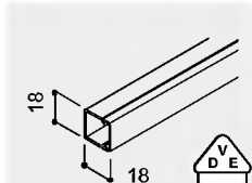
WDK 20020 balení: 60 m hmot.: 0,245 kg/m
