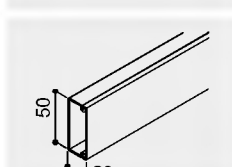
WDK 20050 balení: 24 m hmot.: 0,315 kg/m
