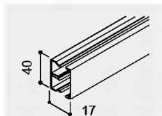
WDK-N 15040 balení: 54 m hmot.: 0,315 kg/m
