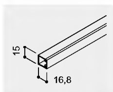
WDK 15015 balení: 60 m hmot.: 0,110 kg/m
