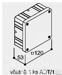
WDK/AK 120 balení: 1 ks hmot.: 0,200 kg/ks
