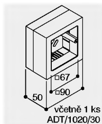
WDK/TS balení: 1 ks hmot.: 0,060 kg/ks
