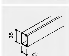
WDK 20035 balení: 28 m hmot.: 0,230 kg/m
