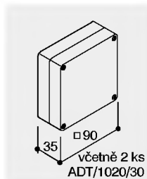
WDK/AK 90 balení: 2 ks hmot.: 0,080 kg/ks
