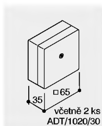
WDK/AK 65 balení: 2 ks hmot.: 0,049 kg/ks.
