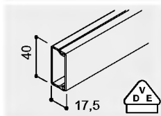
WDK 15040 balení: 28 m hmot.: 0,230 kg/m
