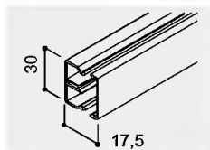
WDK-N 15030 balení: 40 m hmot.: 0,240 kg/m
