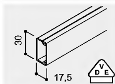
WDK 15030 balení: 40 m hmot.: 0,220 kg/m
