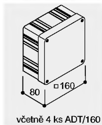
WDK/AK 160 balení: 1 ks hmot.: 0,400 kg/ks
