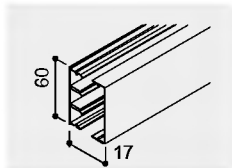
WDK-N 15060 balení: 36 m hmot.: 0,365 kg/m
