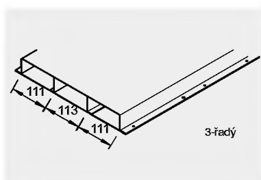
UK 3448-3 balení: 1 ks hmot.: 9,100 kg/m
