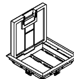
GEE 4/6-5 balení: 1 ks hmot.: 1,217 kg/ks
