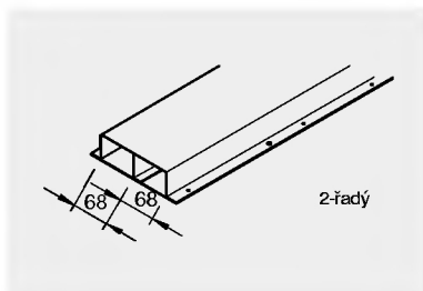
UK 1448-2 balení: 1 ks hmot.: 4,400 kg/m
