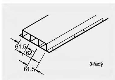
UK 1948-3 balení: 1 ks hmot.: 6,150 kg/m
