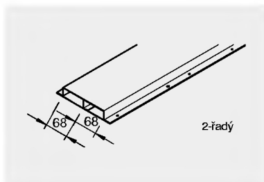
UK 1428-2 balení: 1 ks hmot.: 3,800 kg/m
