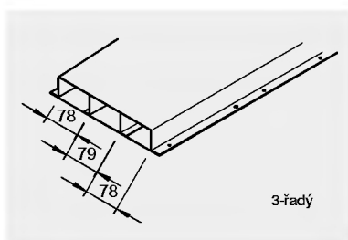
UK 2448-3 balení: 1 ks hmot.: 7,100 kg/m
