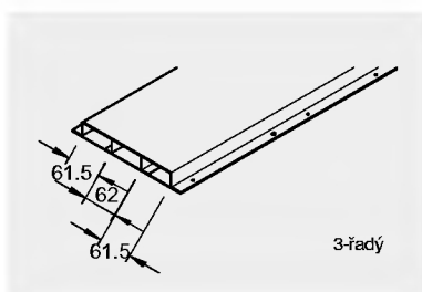
UK 1928-3 balení: 1 ks hmot.: 5,200 kg/m
