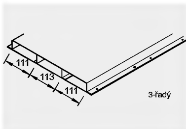
UK 3438-3 balení: 1 ks hmot.: 8,450 kg/m
