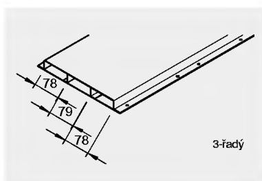
UK 2428-3 balení: 1 ks hmot.: 6,200 kg/m
