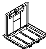
Přístrojová jednotka** s ochranným rámečkem pro podlahovou krytinu tloušťky 5 mm
