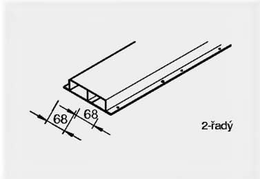
UK 1438-2 balení: 1 ks hmot.: 4,100 kg/m
