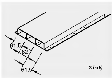
UK 1938-3 balení: 1 ks hmot.: 5,700 kg/m
