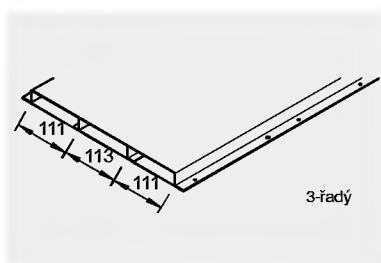
UK 3428-3 balení: 1 ks hmot.: 8,000 kg/m
