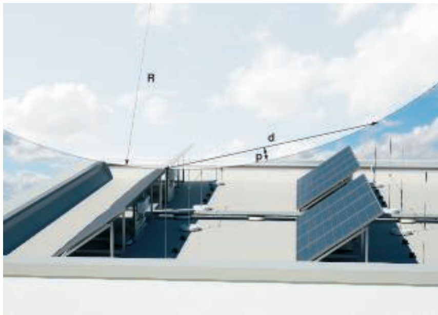
Obr. 1: Metody projektování: Blesková koule (R), metoda bleskové koule s hloubkou průniku (p) a vzdáleností jímacích tyčí (d)
