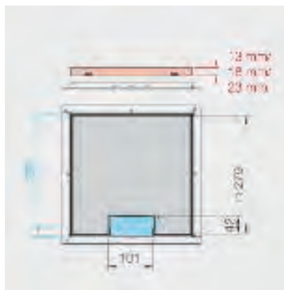
RKS, pro šňůrový vývod, jmenovitá velikost 250-3
