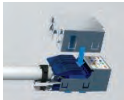
Připojení přístroje – montáž stínicího krytu Stínicí kryt se na modulární zásuvku nasazuje a naklapává shora. Stínicí kryt se používá jen u stíněných modulárních zásuvek.
