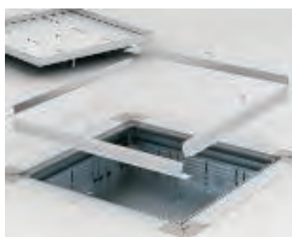
Montáž kazetového rámu na podlahovou krabici Spojte kazetový rám a namontujte jej na tělo krabice (upevňovací šrouby jsou součástí dodávky).
