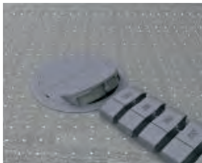
Vývod vedení pro dvojitou podlahu Vývod vedení se šňůrovým vývodem pro použití v podlahách se suchou údržbou. Ohebný kanál se upevňuje přímo k vývodu.
