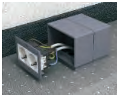
Montáž zásuvky do přístrojového nástavce Přístroj Modul 45 před připojením vedení nasklapněte do krytu.
