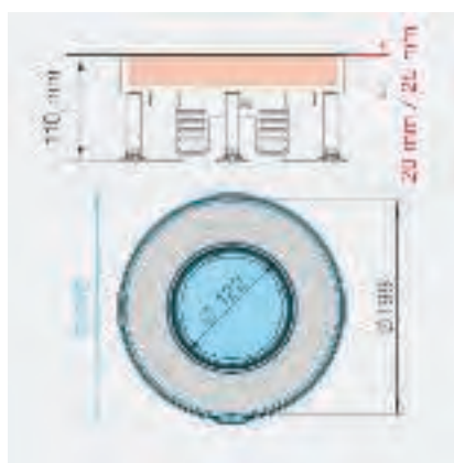
RKFR 2, pro tubus, jmenovitá velikost R4
