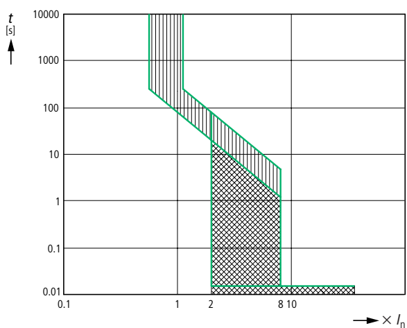
IZM...-A... Ochrana rozvodů
