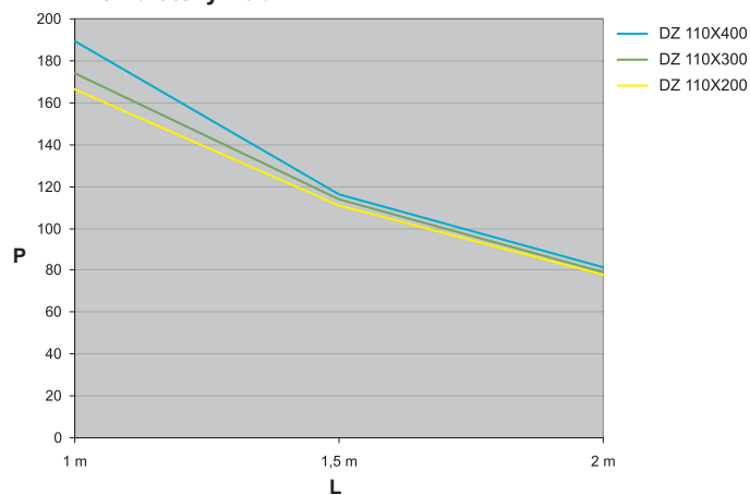
110 - drátěný žlab
