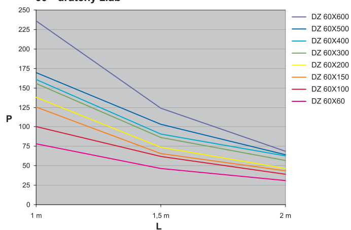
60 - drátěný žlab
