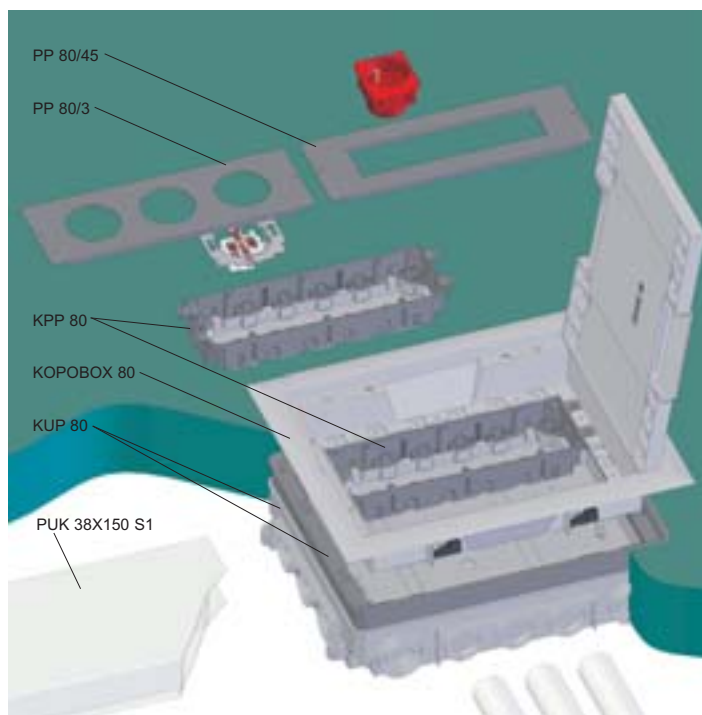
KOPOBOX 80 - sestava
