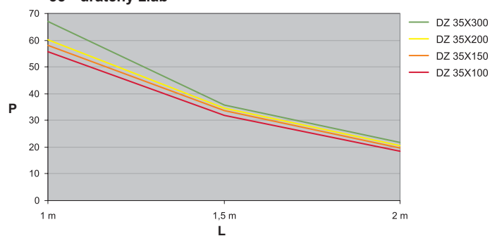
35 - drátěný žlab
