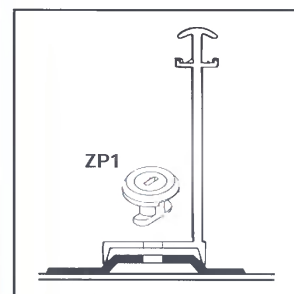
SEP-E detail montáže
