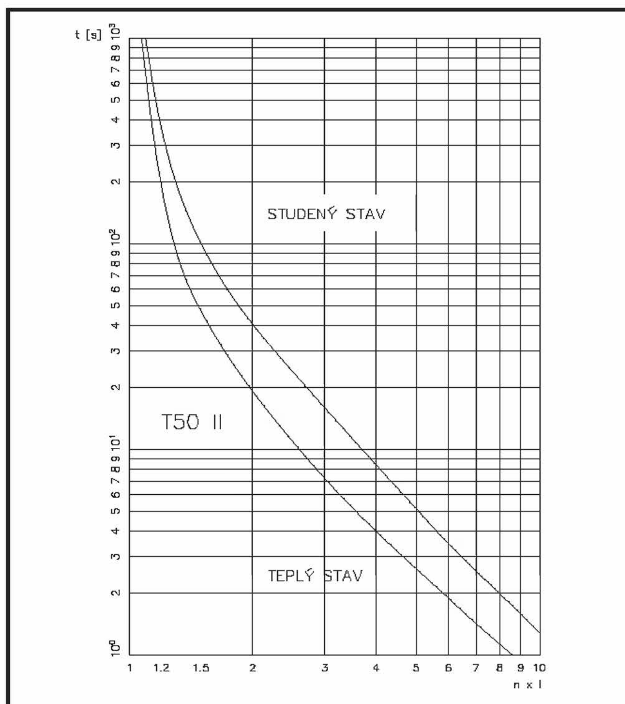
Charakteristika T50 I – dvoupólová – vypínací třída 10 A
