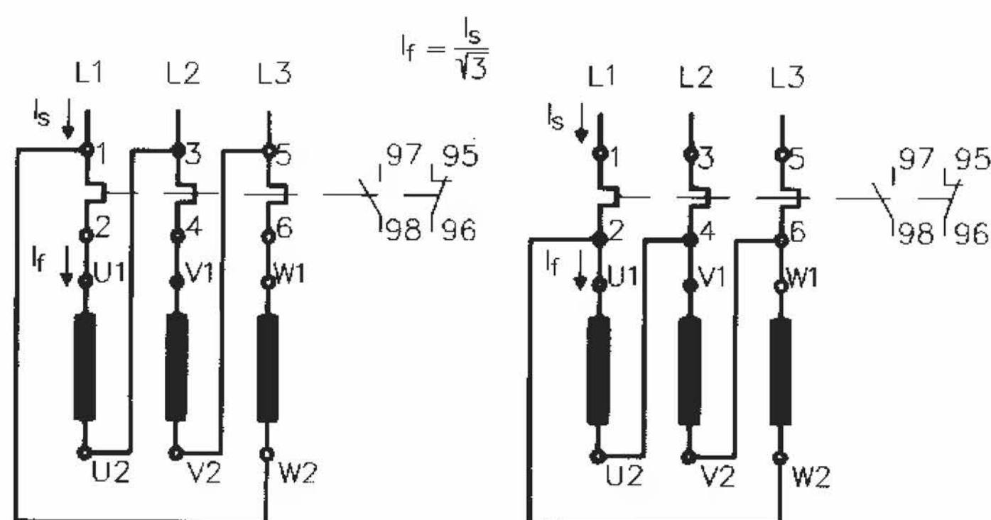
Relé a motor v zapojení do trojúhelníku
