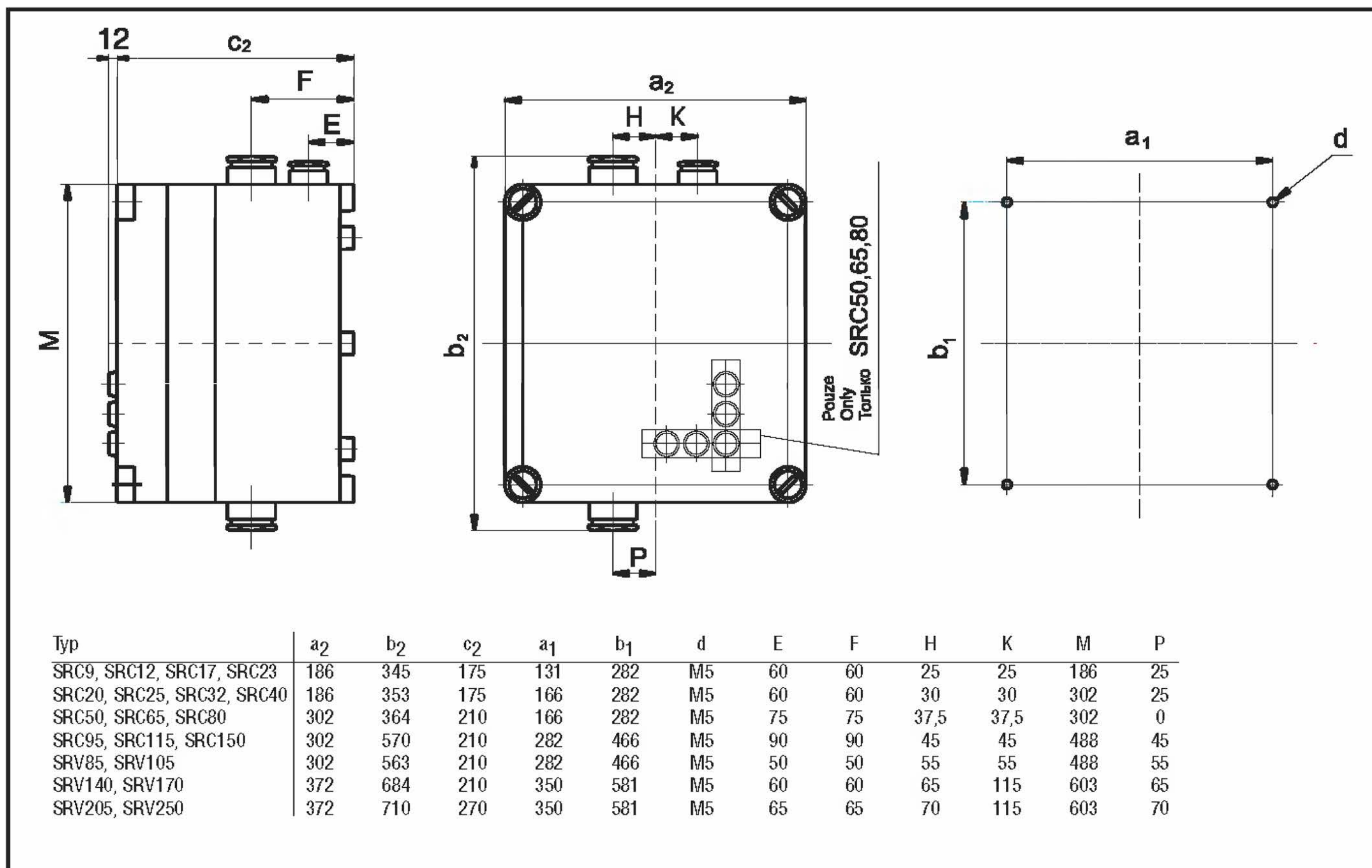
Rozměrový výkres reverzačních spouštěčů SRC, SRV (IP65)
