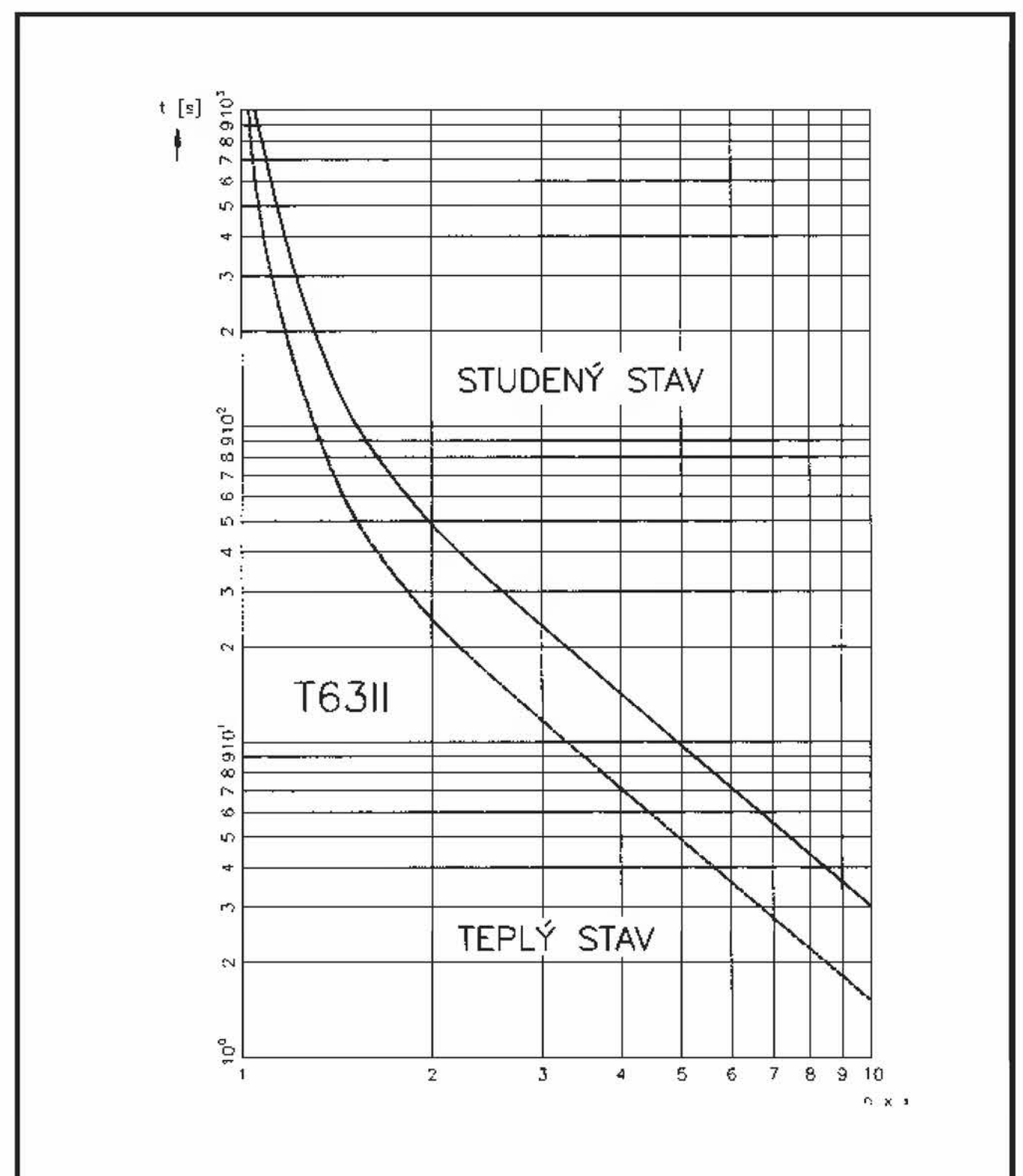
Charakteristika T63 II – dvoupólová – vypínací třída 20
