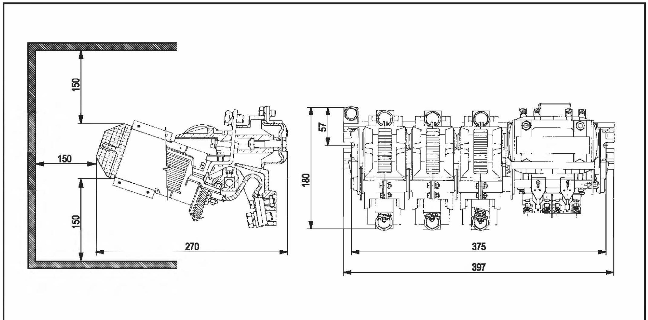
Rozměrový výkres stykače VH400
