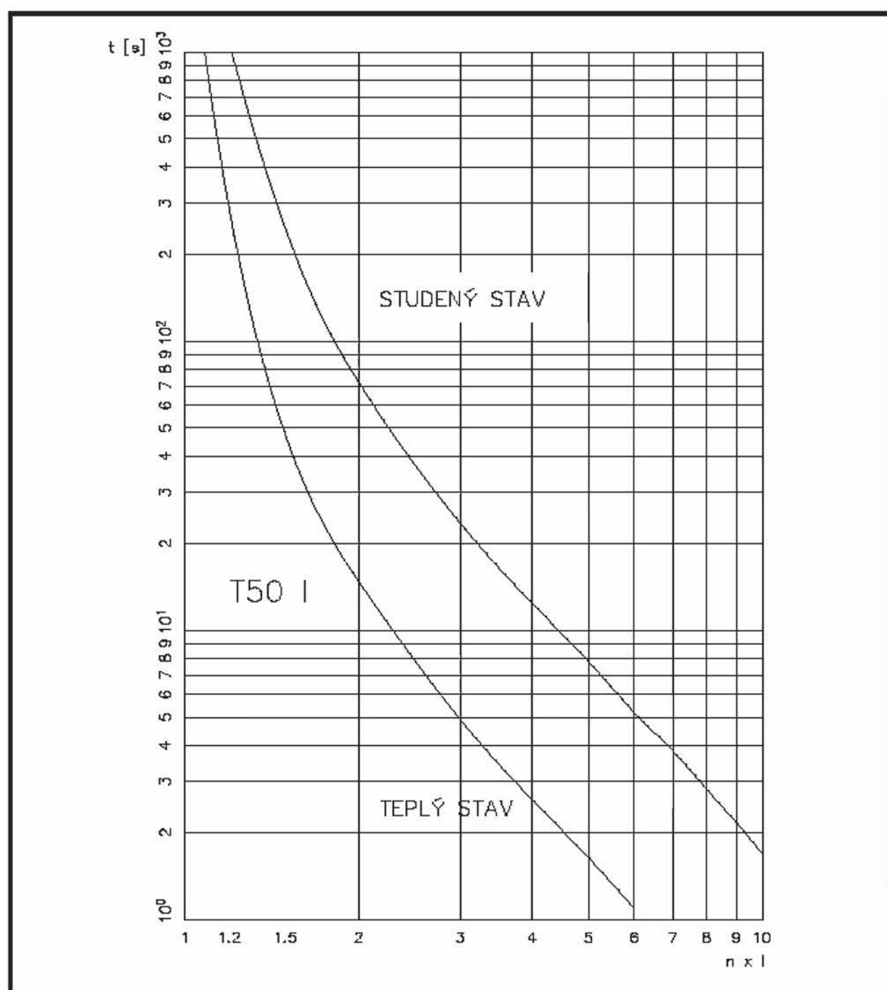
Charakteristika T50 I – trojpólová – vypínací třída 10 A
