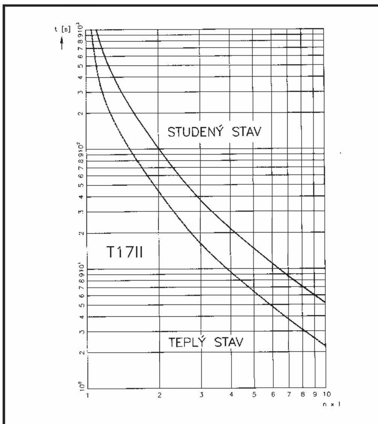
Charakteristika T17 II – trojpólová – vypínací třída 20
