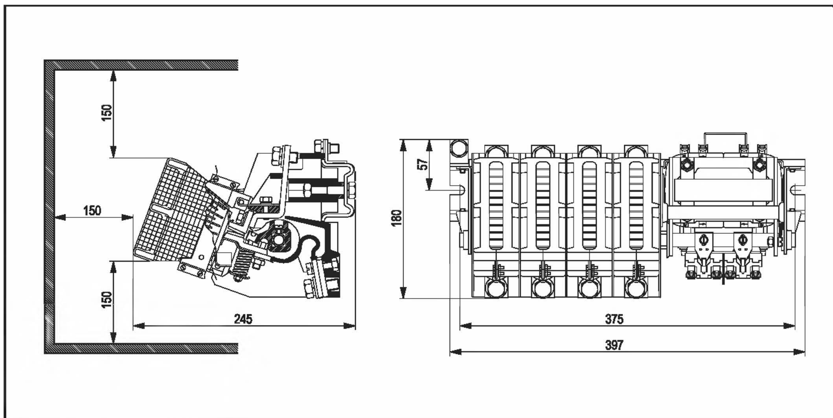
Rozměrový výkres stykače VH250D0.4, VH440.4
