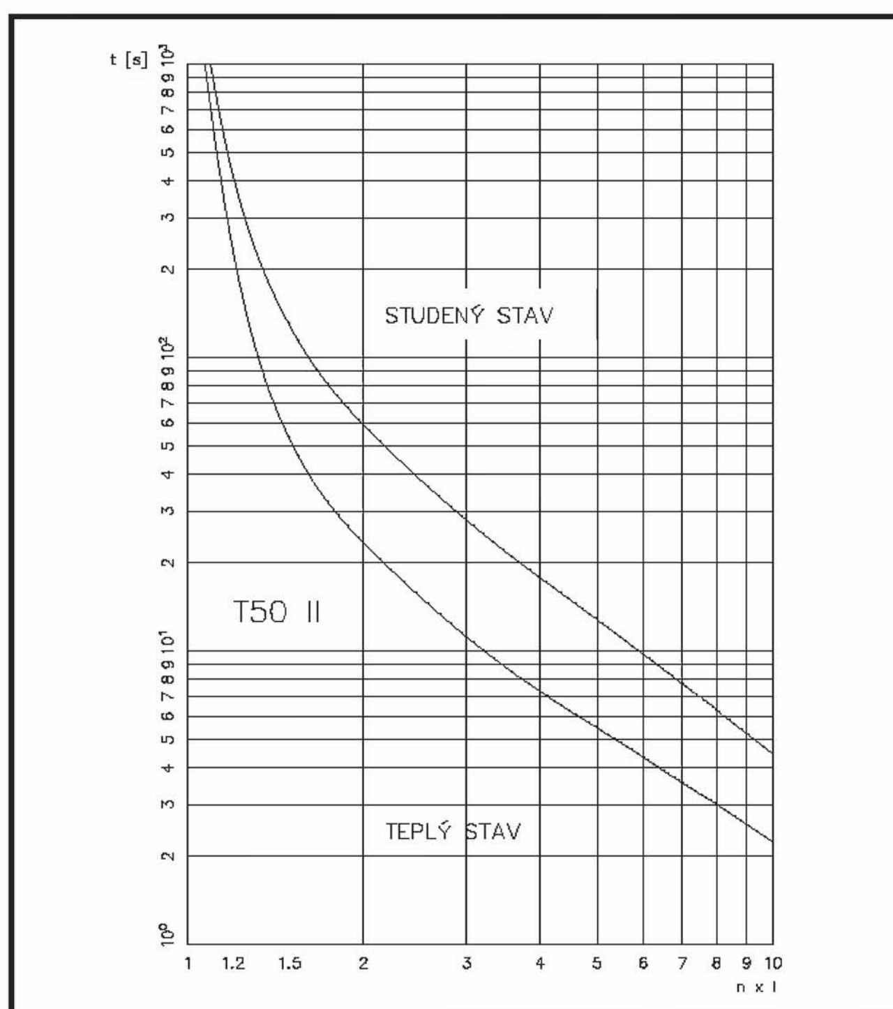
Charakteristika T50 II – dvoupólová – vypínací třída 20
