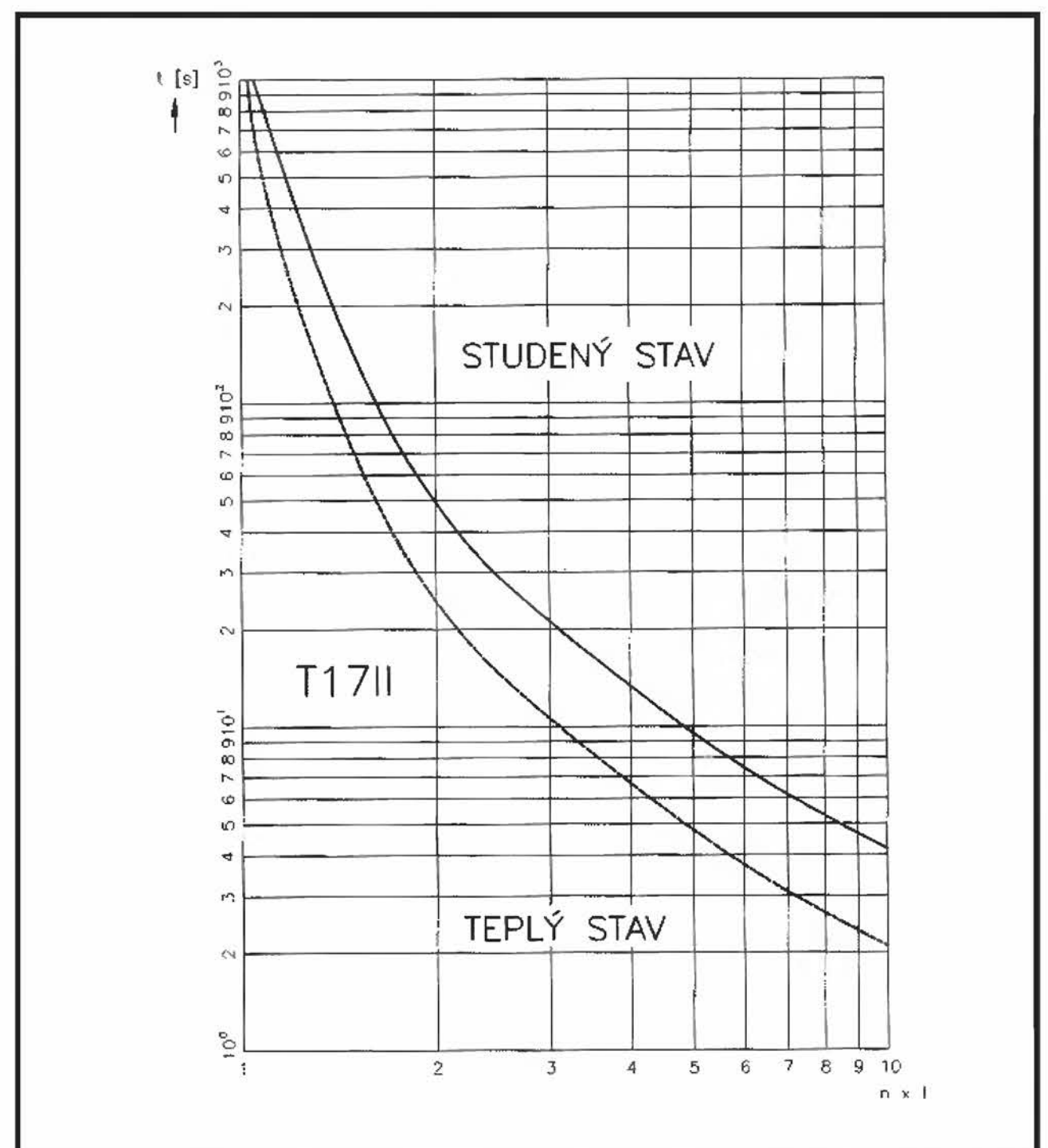
Charakteristika T17 II – dvoupólová – vypínací třída 20
