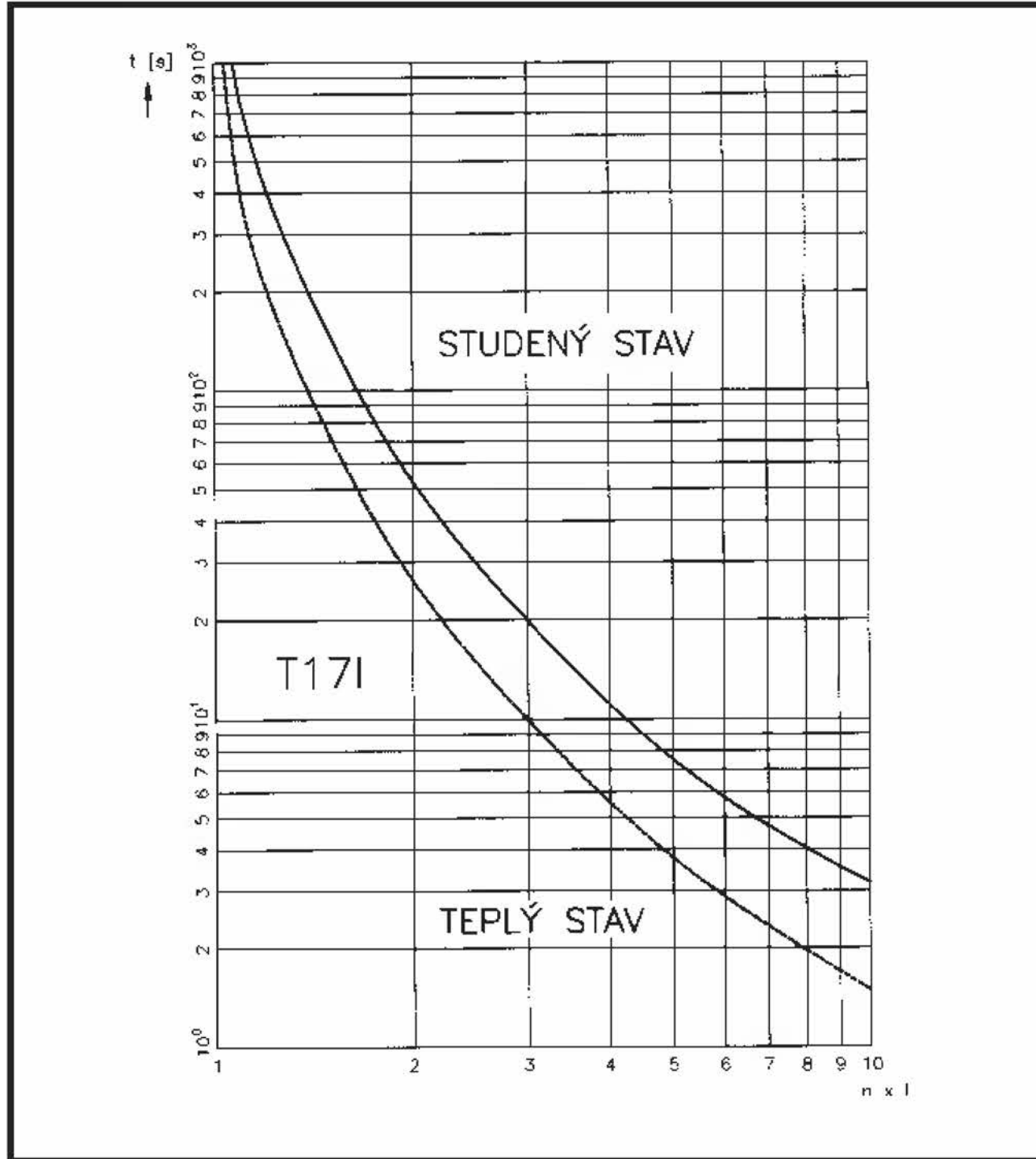
Charakteristika T17 I – trojpólová – vypínací třída 10 A
