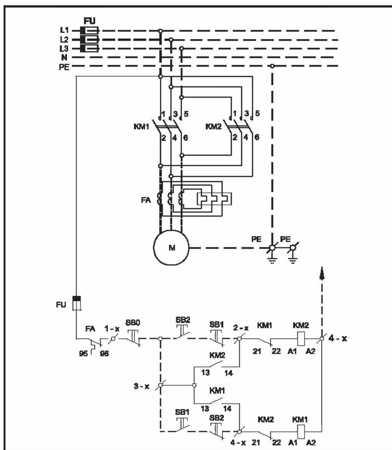
Schéma zapojení reverzačních spouštěčů SRC95, 115, 150, SRV s jisticí soupravou
