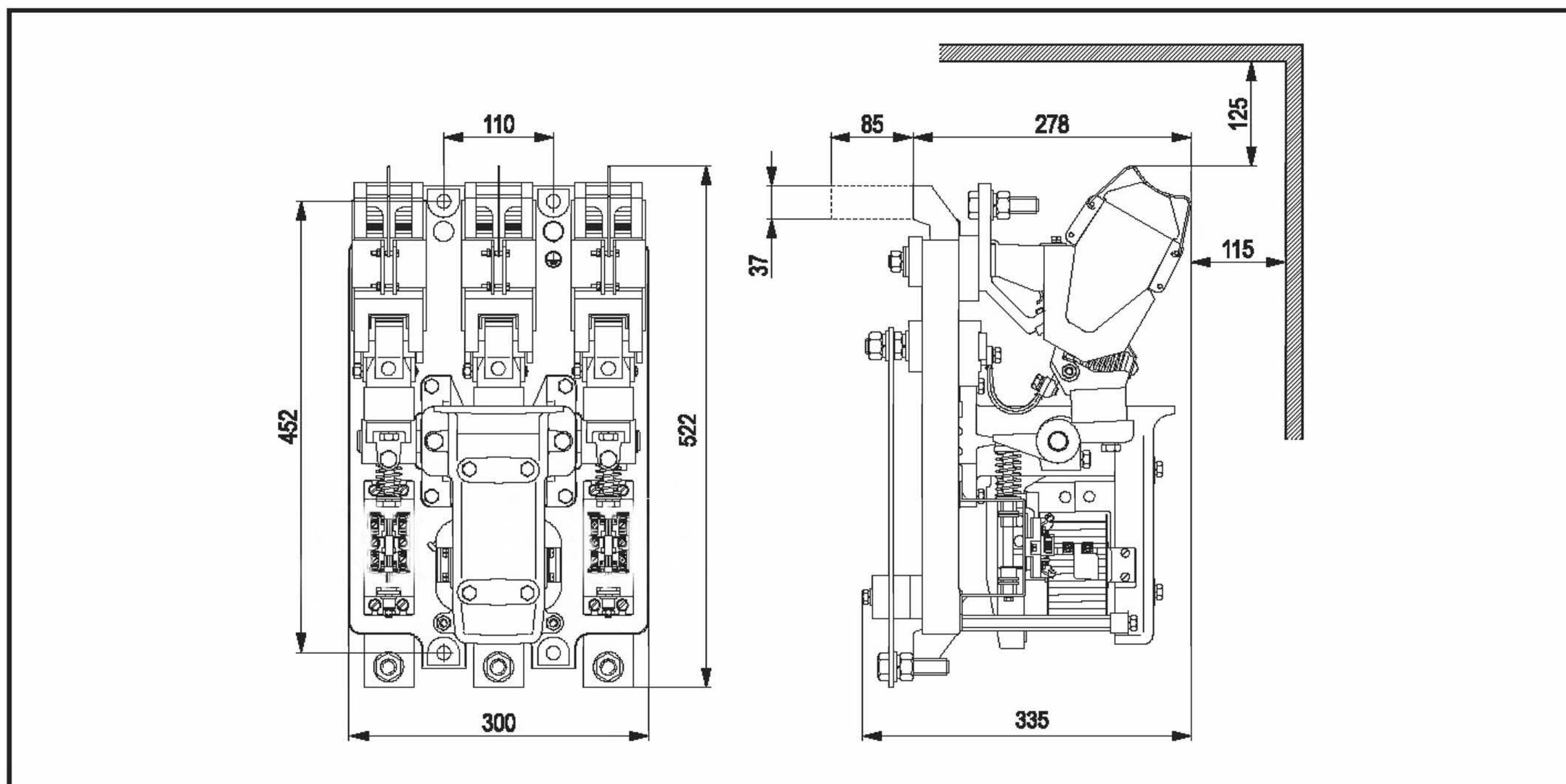
Rozměrový výkres stykače V53D, VD630, VD1000
