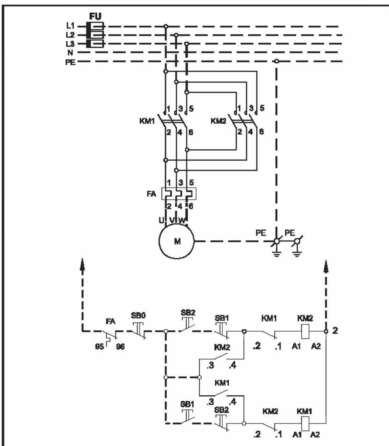
Schéma zapojení reverzačních spouštěčů SRC 9..80 s jisticím relé
