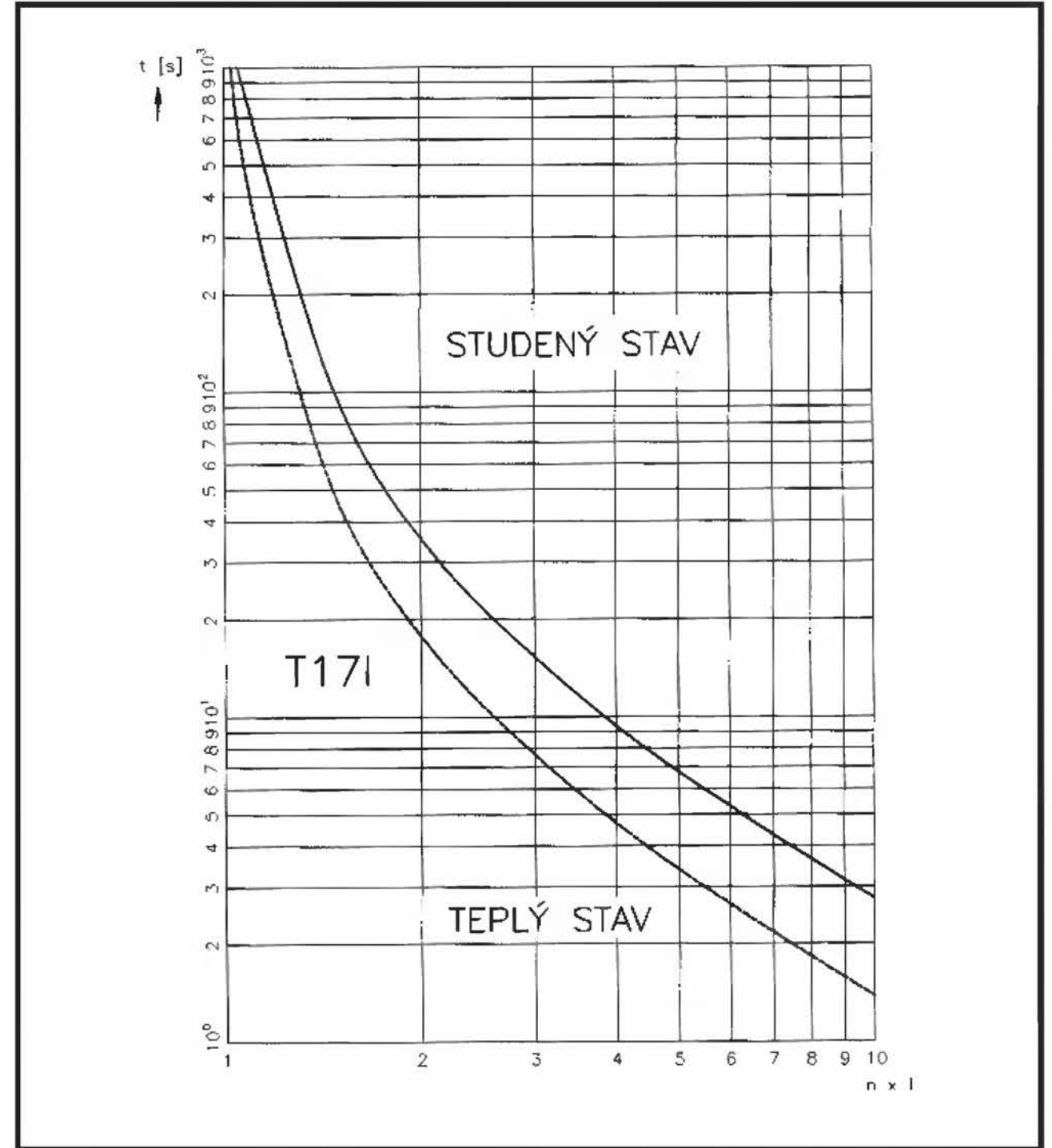
Charakteristika T17 I – dvoupólová – vypínací třída 10 A
