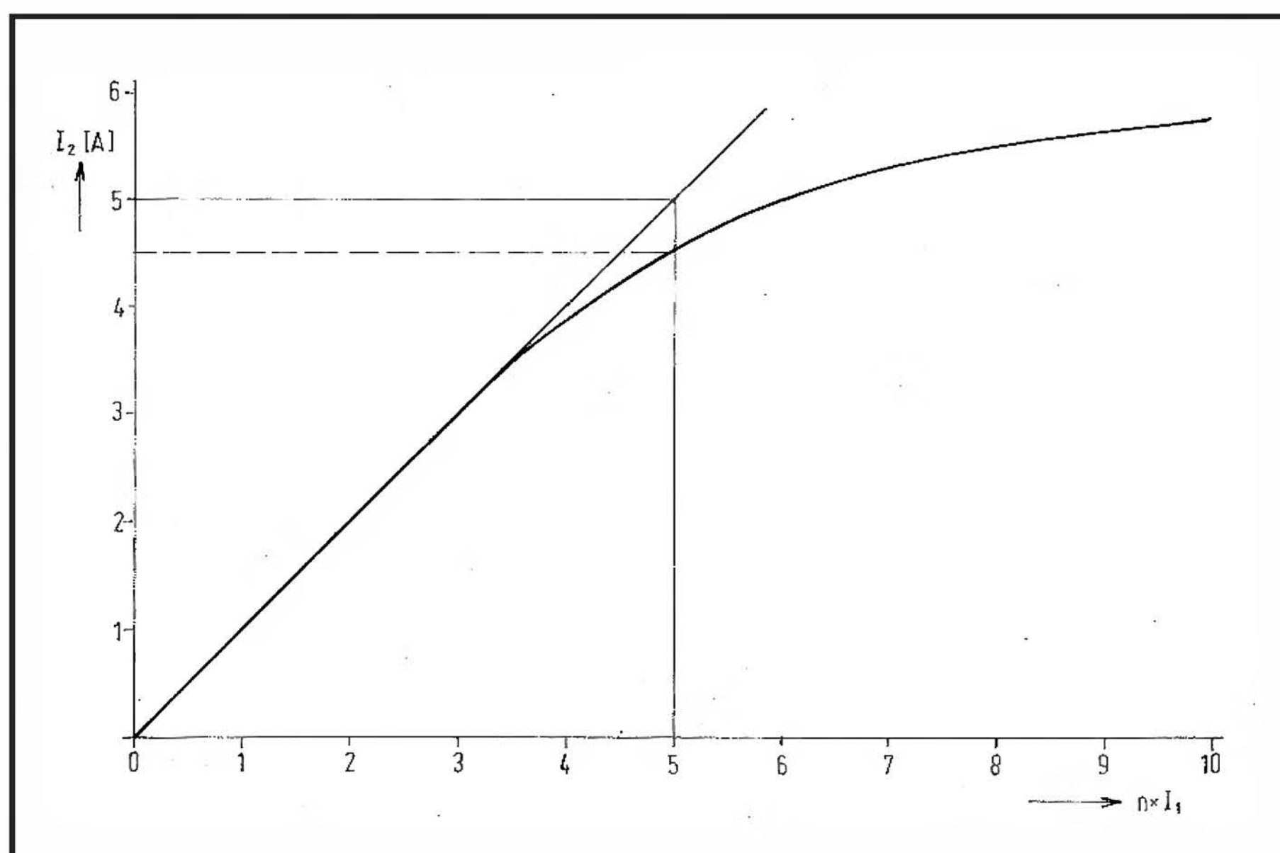
Převodní charakteristika jistícího transformátoru M
