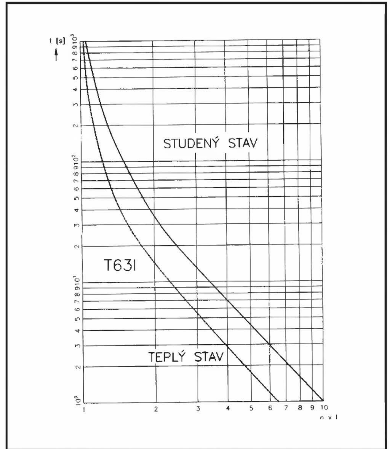
Charakteristika T63 I – dvoupólová – vypínací třída 10 A
