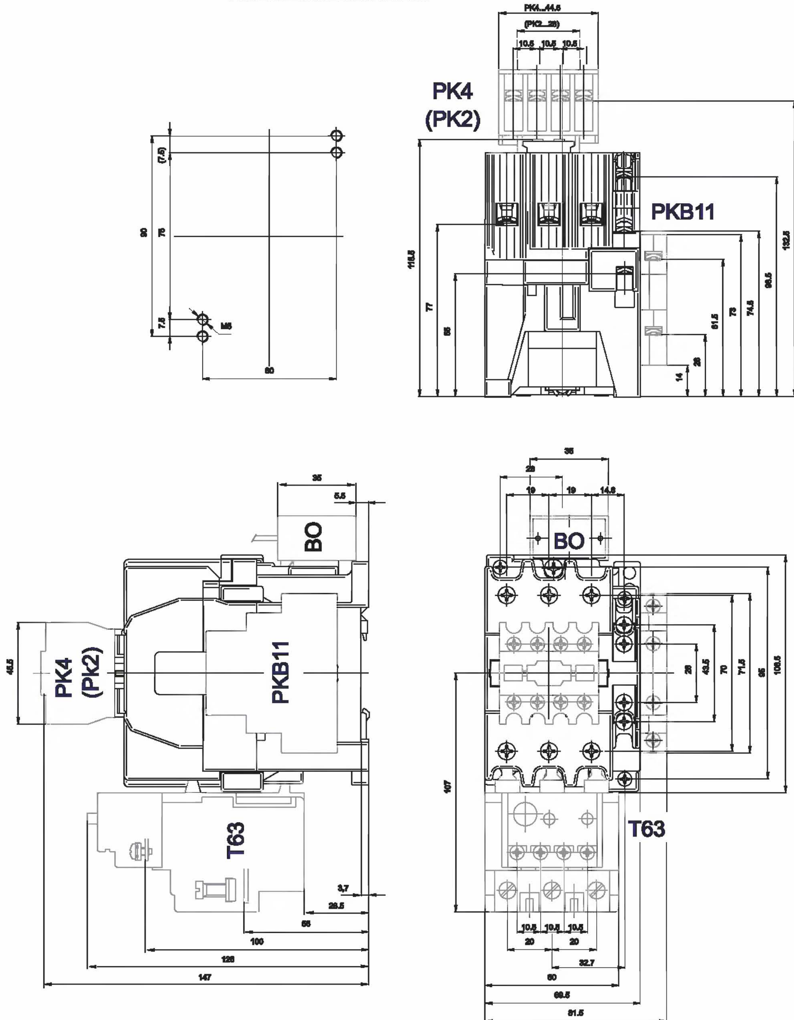
POHLED BEZ NASAZENÉHO RELÉ T63
