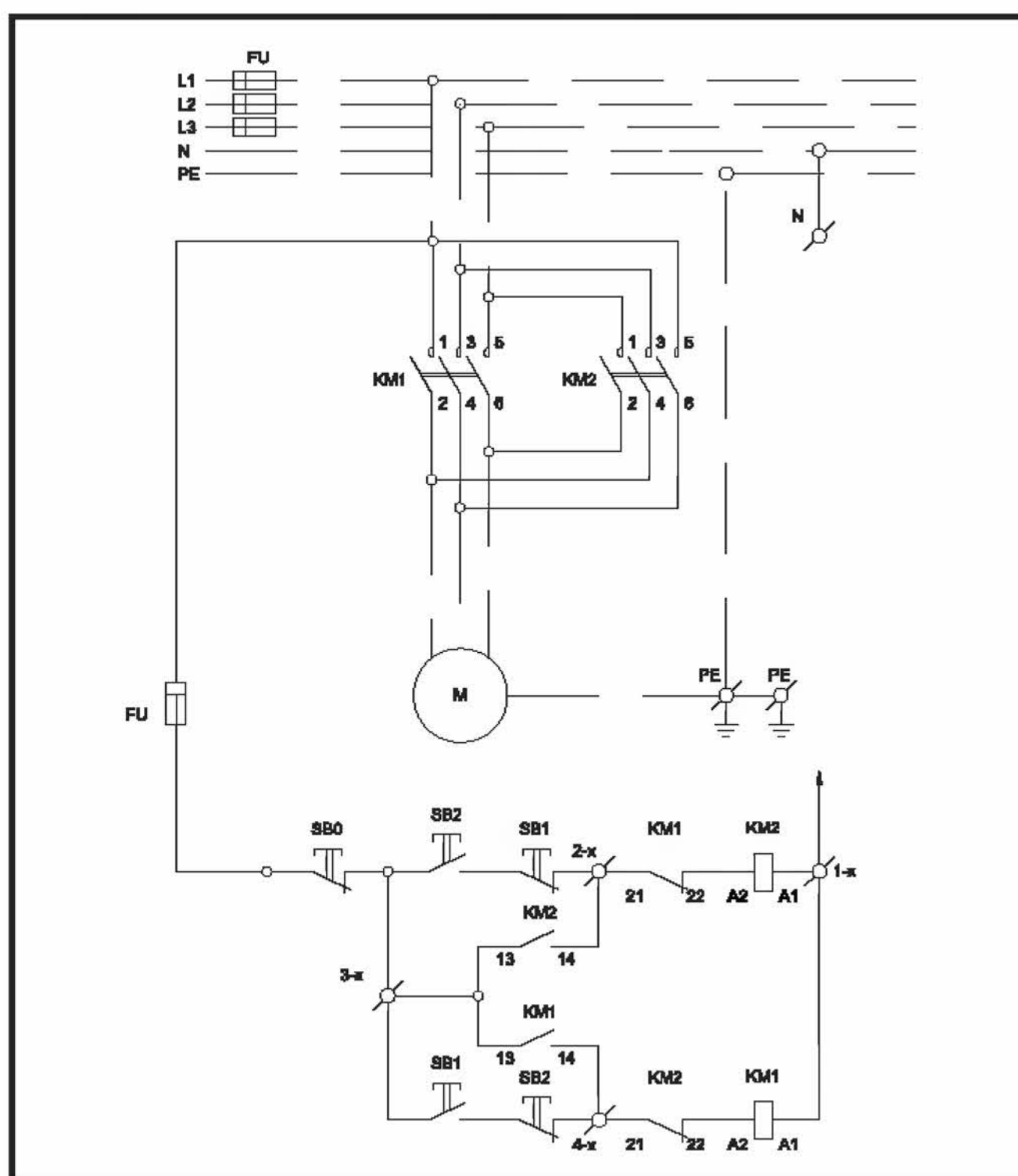
Schéma zapojení SRV85, 105, 140, 170, 205, 250
