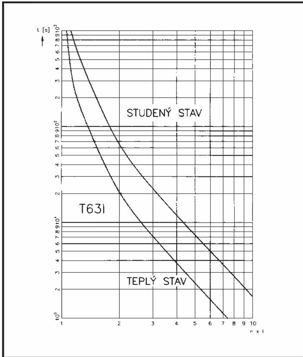
Charakteristika T63 I – trojpólová – vypínací třída 10 A
