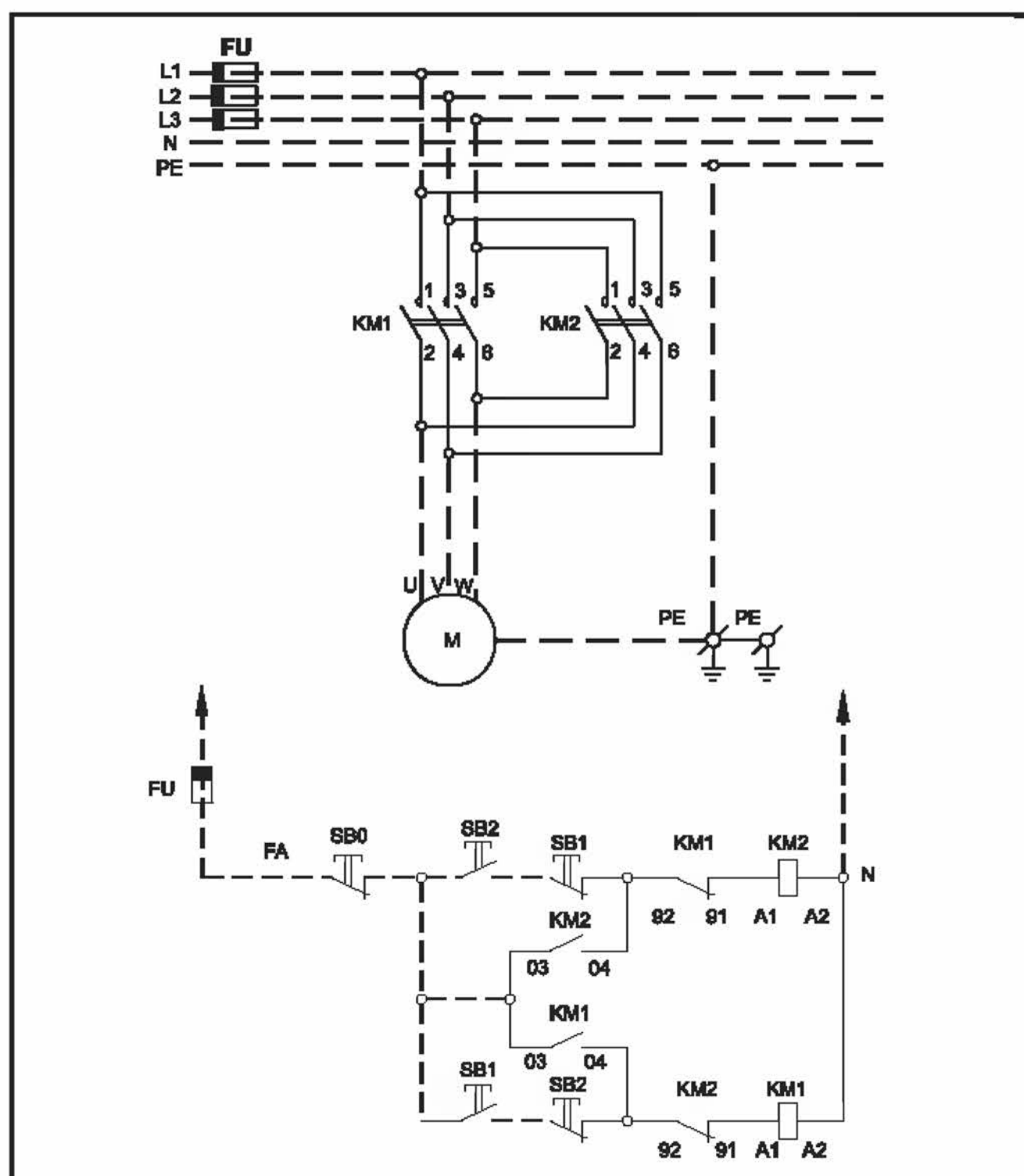
Schéma zapojení reverzačních spouštěčů SRC bez jištění
