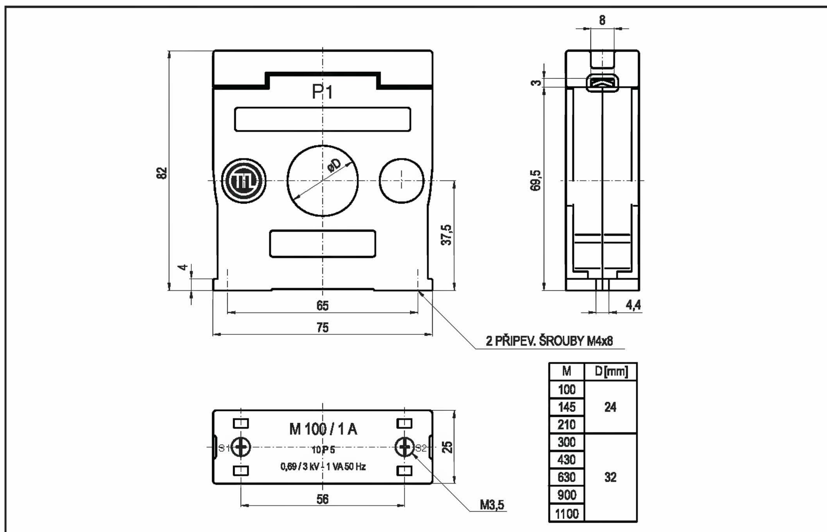
Rozměrový výkres jistícího transformátoru M
