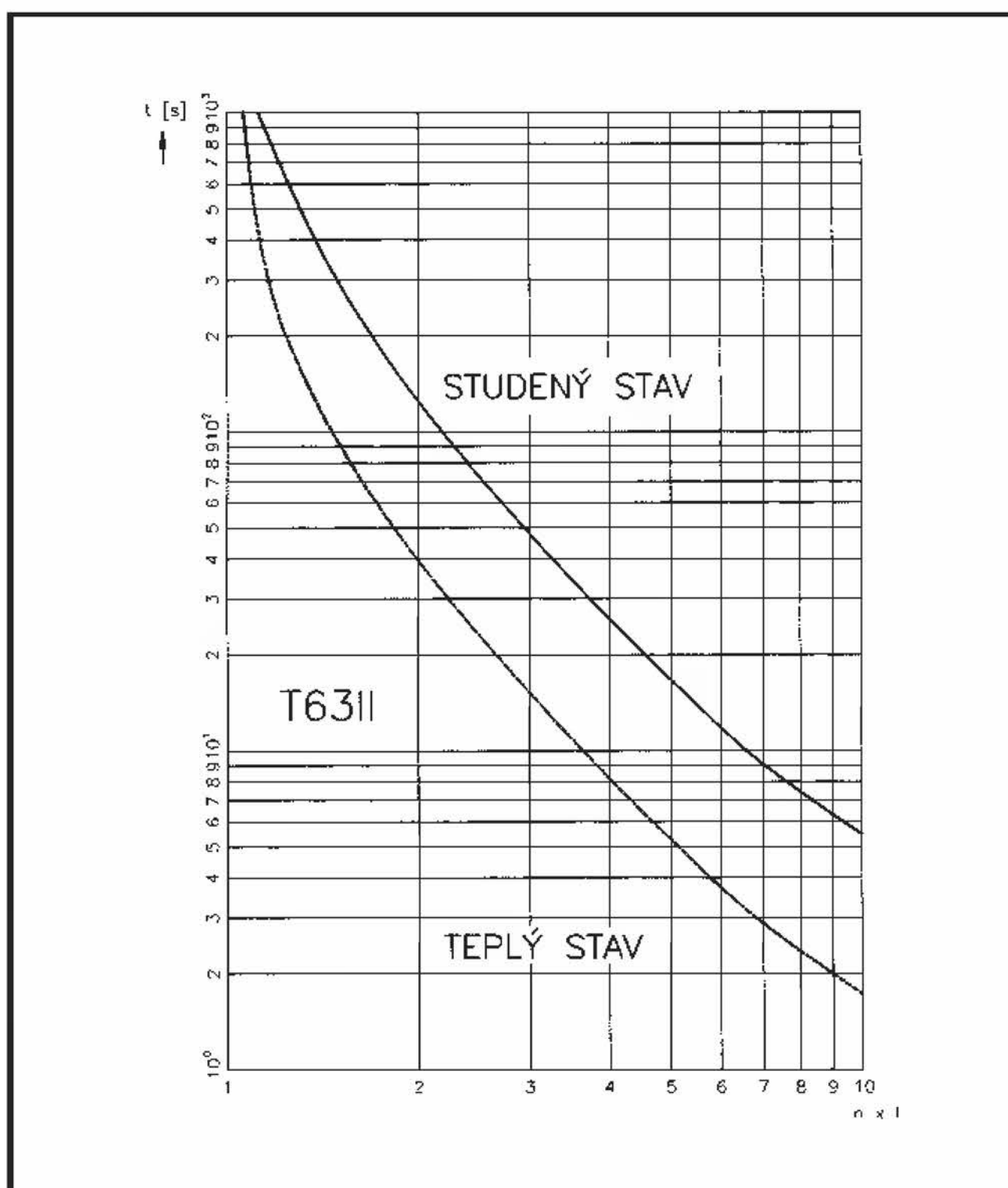
Charakteristika T63 II – trojpólová – vypínací třída 20
