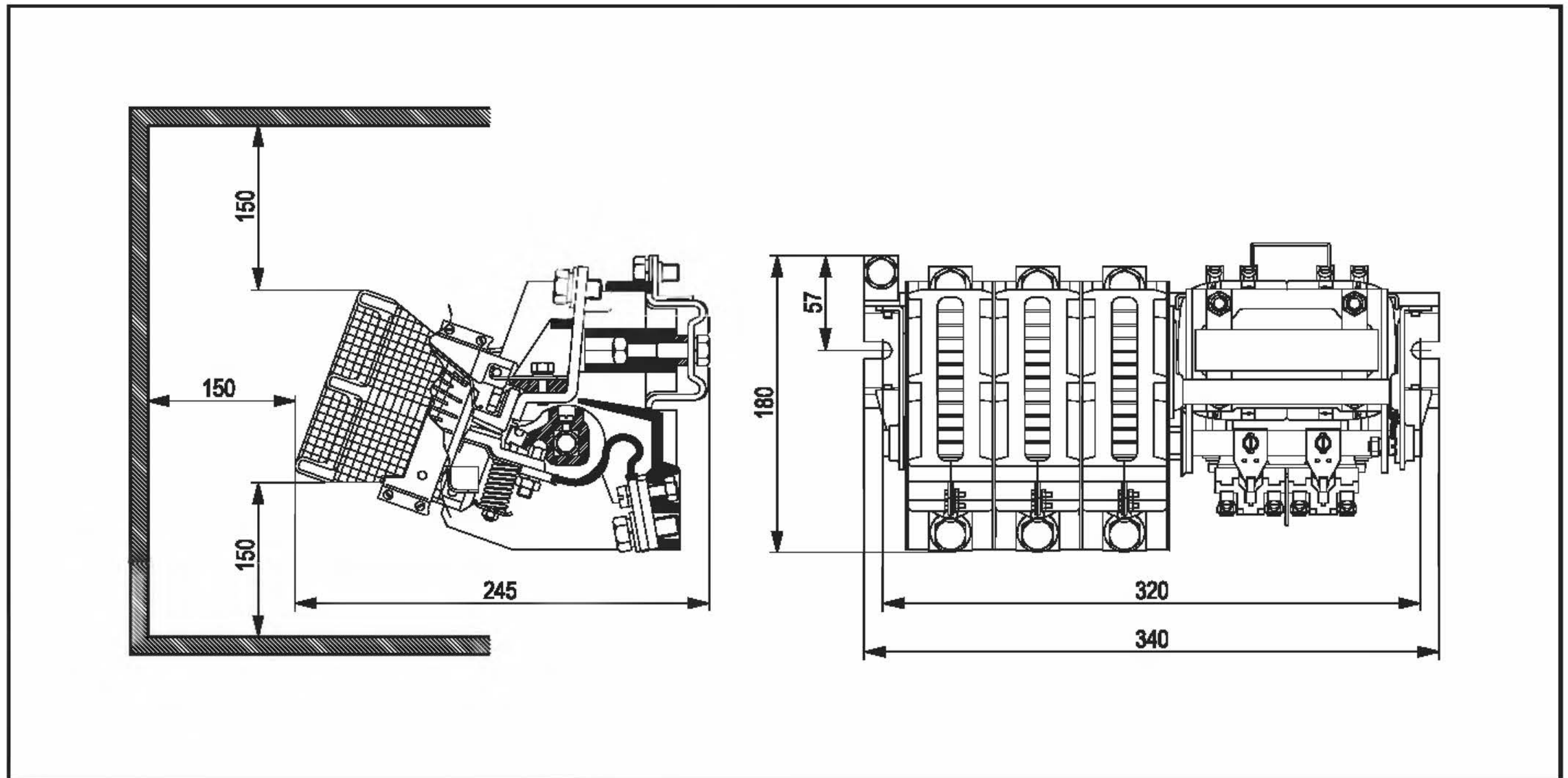
Rozměrový výkres stykače VH250D0, VH440
