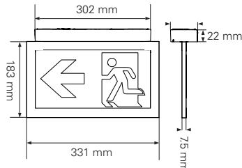
Montáž na povrch stropu
