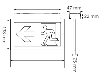
Montáž na povrch stropu
