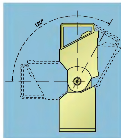
Nastavitelná hlava pro směrování světelného paprsku
