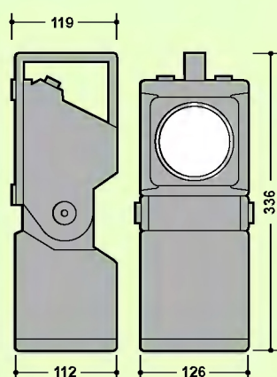
ROZMĚRY (mm)
